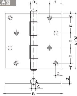
寸法図
