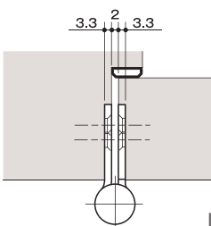
取付図
