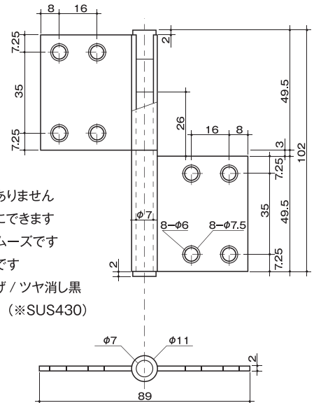
寸法図
