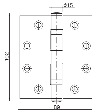
寸法図
