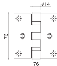
寸法図
