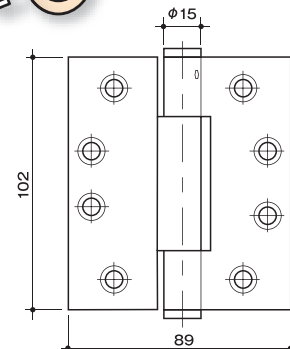
寸法図
