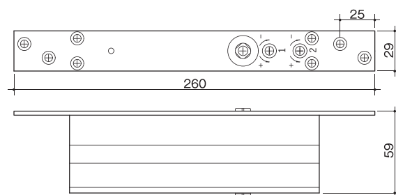
寸法図 本体
