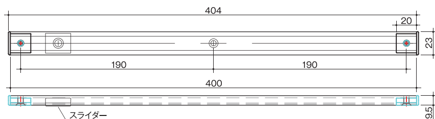
寸法図 レール
