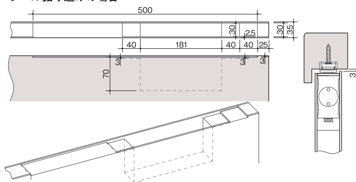
レール掘り込みの場合
