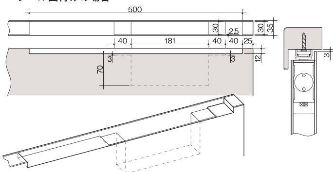
レール面付けの場合
